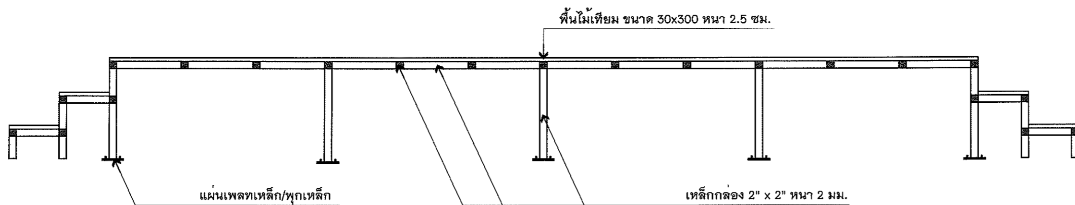
รูปตัด B - B
